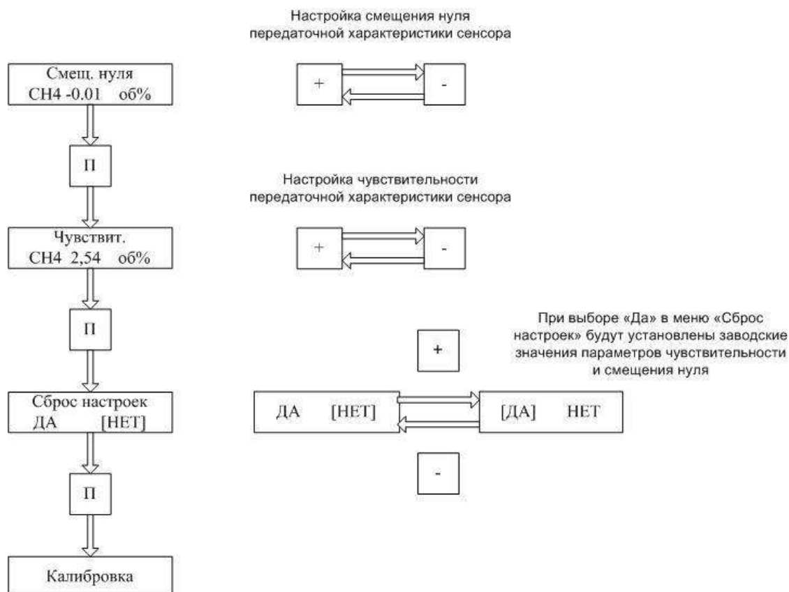
Рисунок 5 – Меню калибровки преобразователей ПГТ-903М19, ПГЭ-903М19
